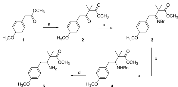
Scheme 1. Reagents: (a) Zn, methyl 2-bromoisobutyrate, THF; (b) TiCl 4 , benzylamine, CH 2 Cl 2 ; (c) NaCNBH 3 ; (d) HCO 2 NH 4 , Pd/C, MeOH.
